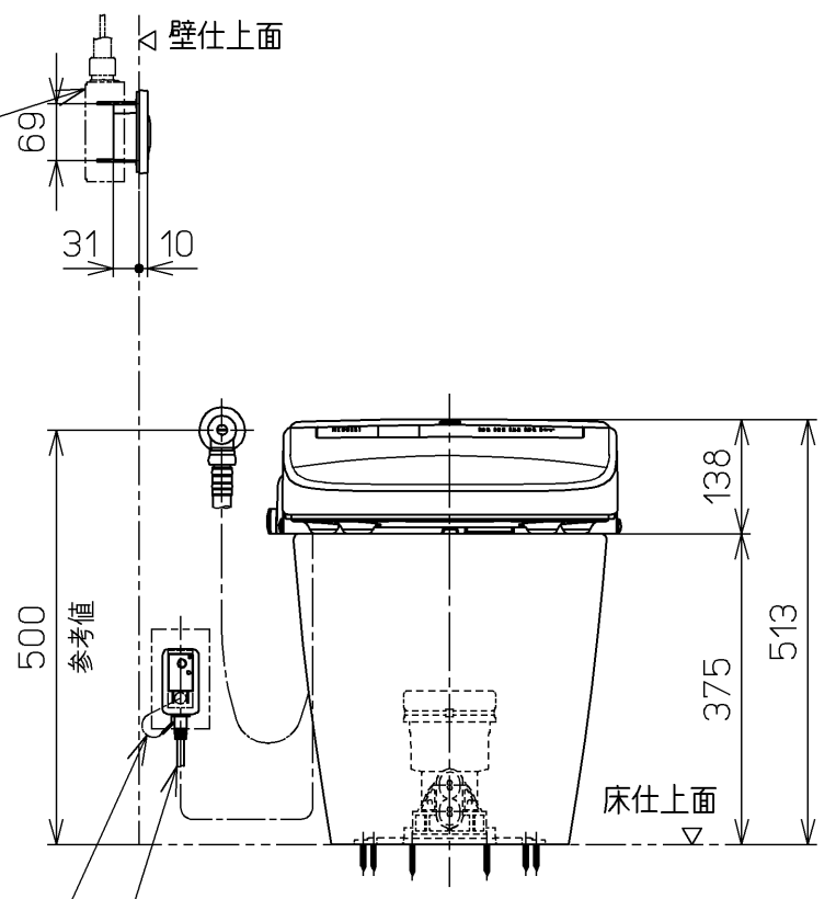
壁給水仕様の場合
